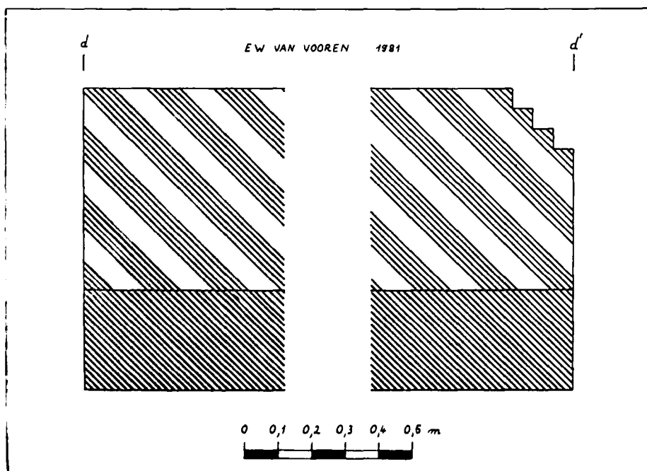
Fig. 8a - Sub-detailplan X 4c : langsdoorsnede van de noordelijke grondvesten.
