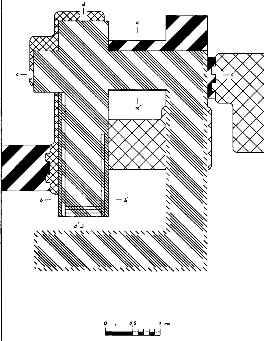
Fig. 6 - Detailplan X 4 : de zgn. onvoltooide hoeve wordt gerealiseerd; gezien de breedte van het zuidelijk en het oostelijk fundament nergens kan worden uit afgeleid is de voorstelling overeenkomstig. Opmerkelijk overigens is het niet gesloten grondplan.
