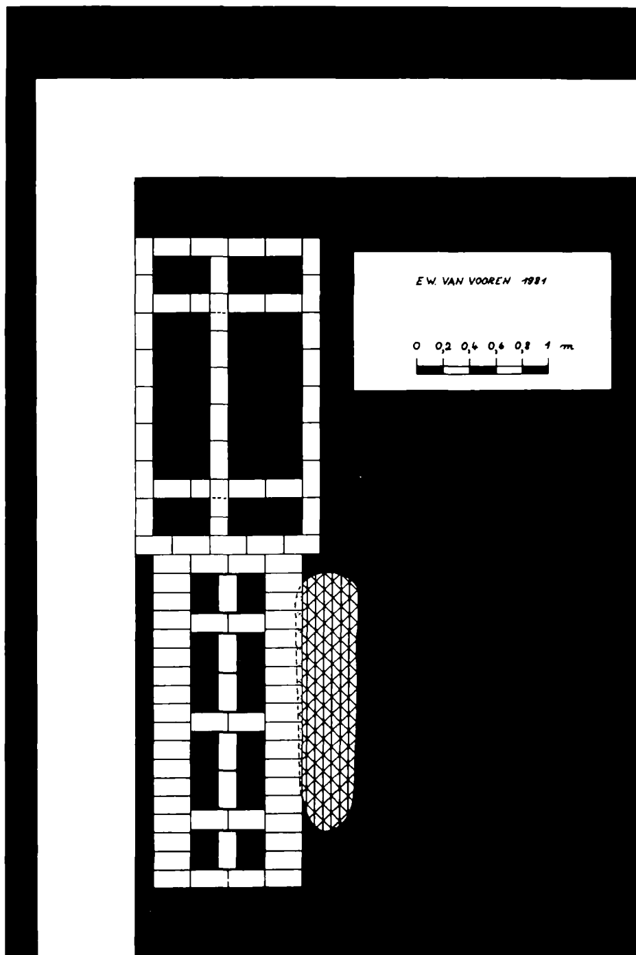
Fig. 13 - Detailplan Y 5 : grafkelder I 1 ondergaat een tweedeling waardoor grafkelder I 2 N en I 2 Z ontstaan.
