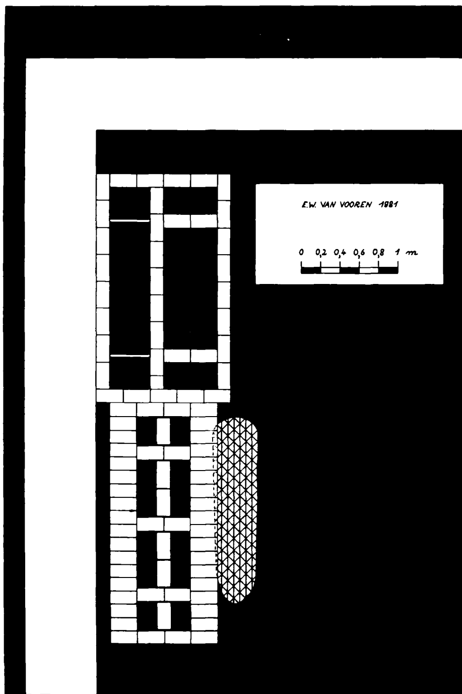
Fig. 14 - Detailplan Y 6 : de bakstenen substructuur van grafkelder I 2 N wordt vervangen door een houten substructuur.
