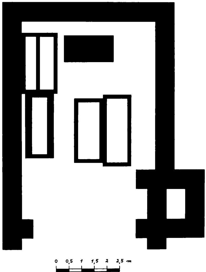
Fig. 19 - Synthetisch reconstructieplan van de eerste bouwtoestand van het koor (enkel de baksteenstructuren zijn weerhouden).
