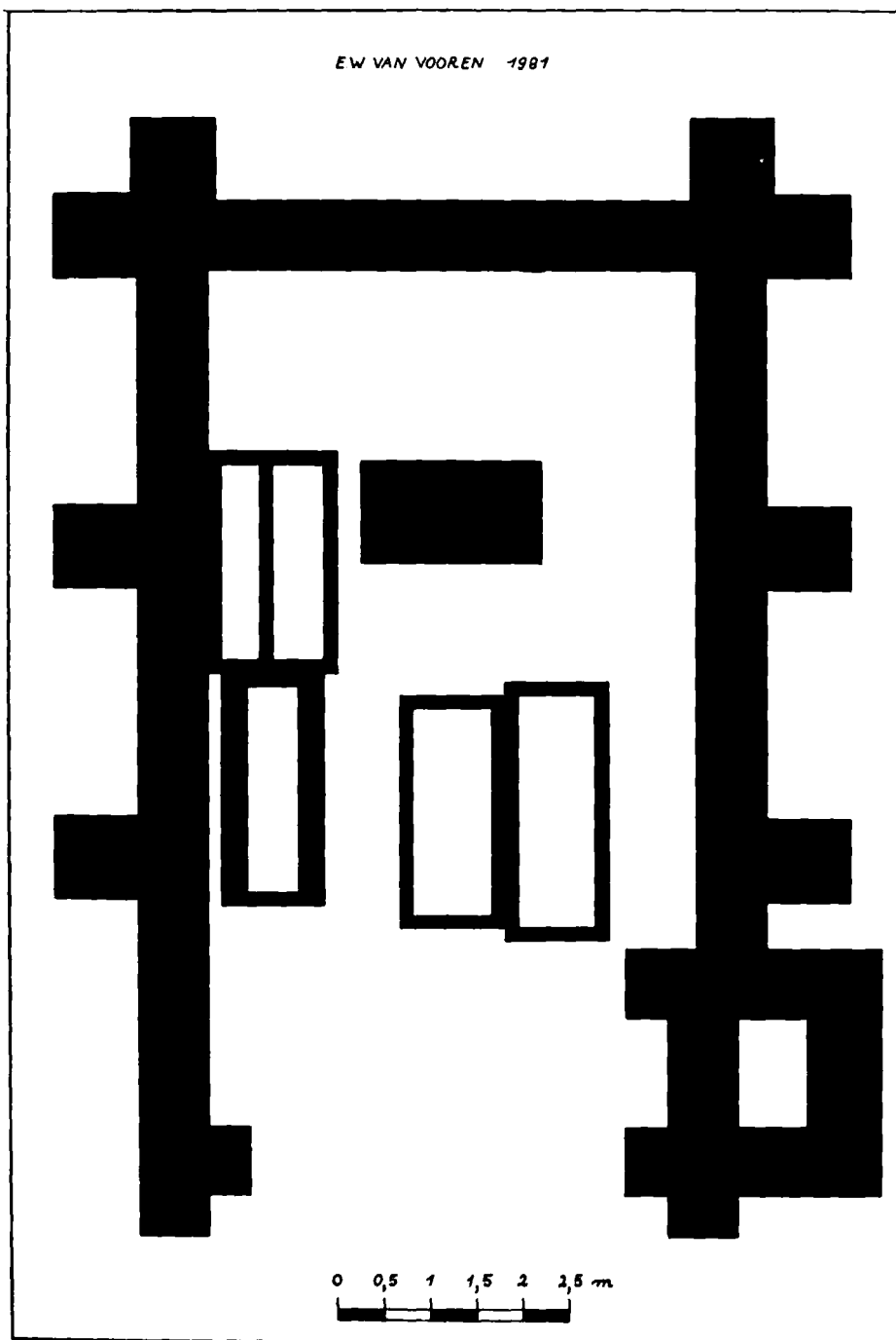
Fig. 20 - Synthetisch reconstructieplan van de tweede bouwtoestand van het koor (enkel de baksteenstructuren zijn weerhouden).
