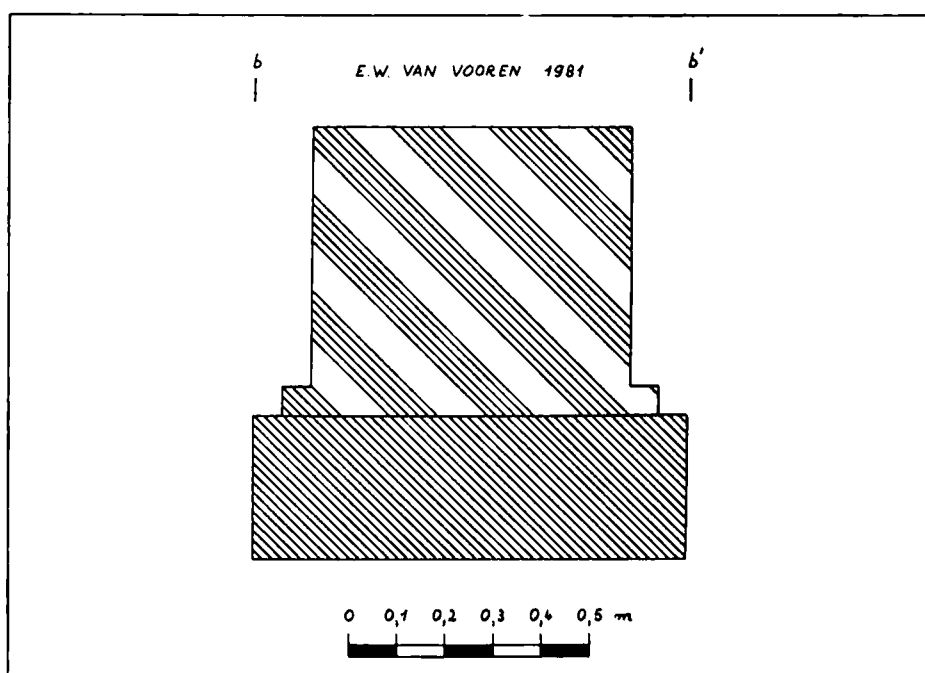
Fig. 7a - Sub-detailplan X 4a : dwarsdoorsnede van de noordelijke grondvesten.
