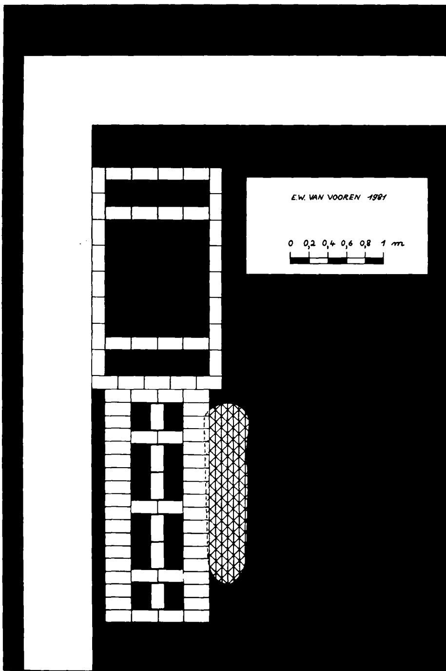
Fig. 12 - Detailplan Y 4 : grafkelder II wordt tegen de westelijke wand van grafkelder I 1 gebouwd.
