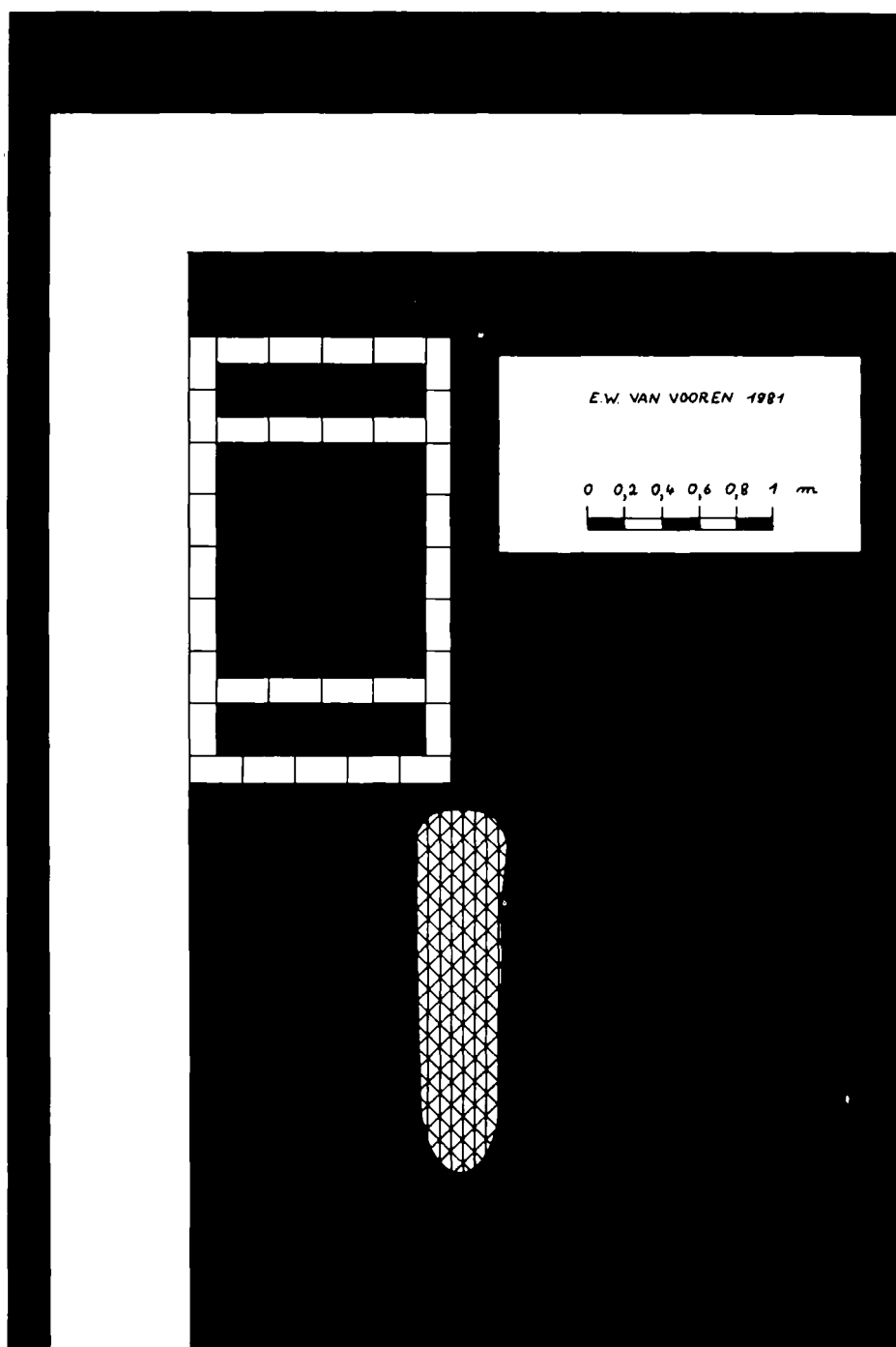
Fig. 11 - Detailplan Y 3 : grafkelder I 1 wordt tegen het fundament van de noordelijke koormuur gebouwd.
