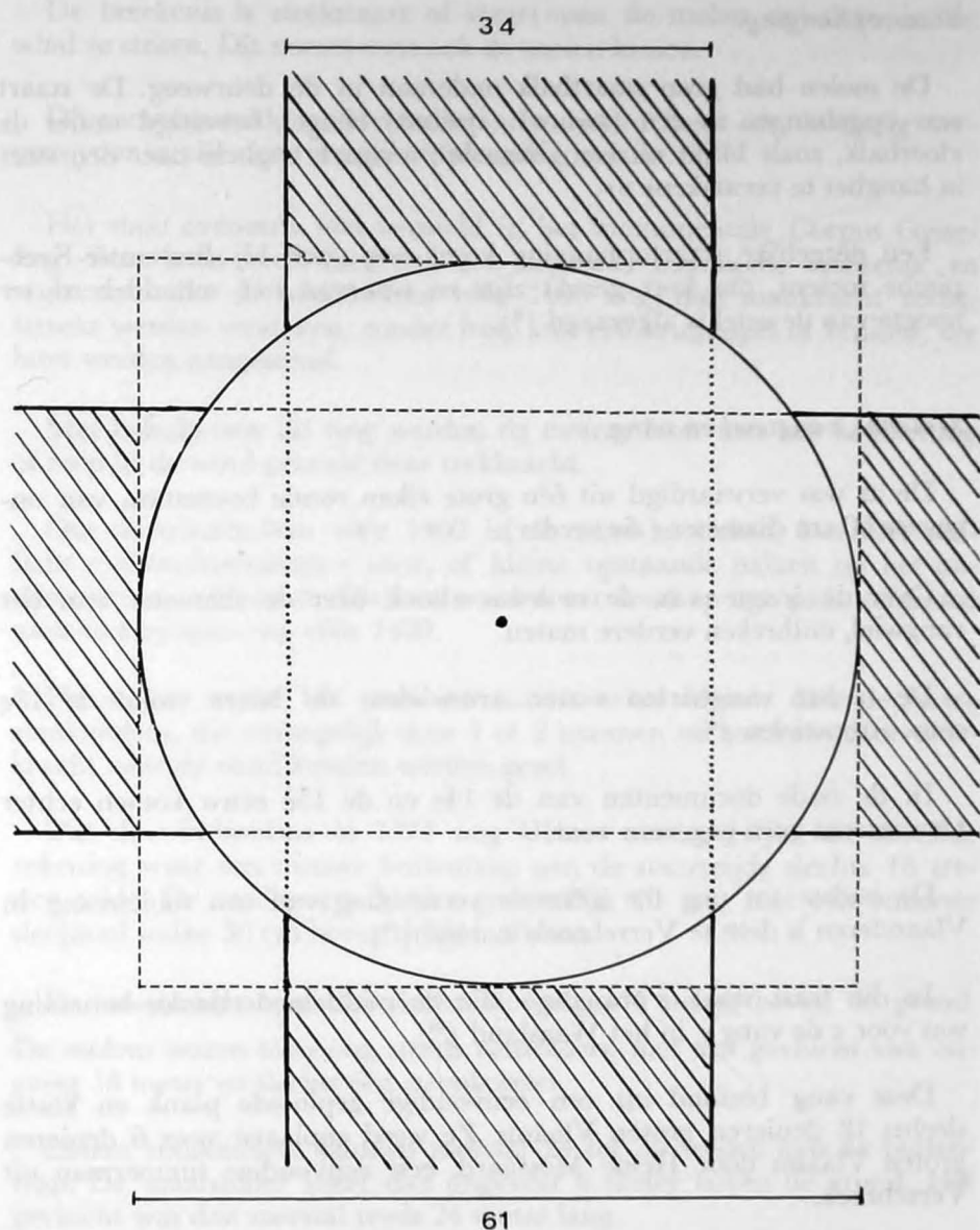
Fig. 6 : Berekende maten in cm. van de houten assekop en pestelbalken van de windmolen te Aalter in 1375.
