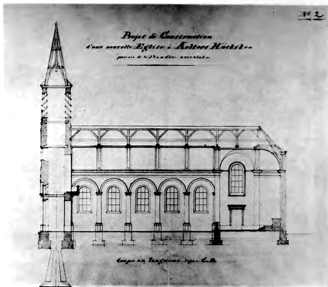
9. Overlangse doorsnede volgens het ontwerp van Suys.
