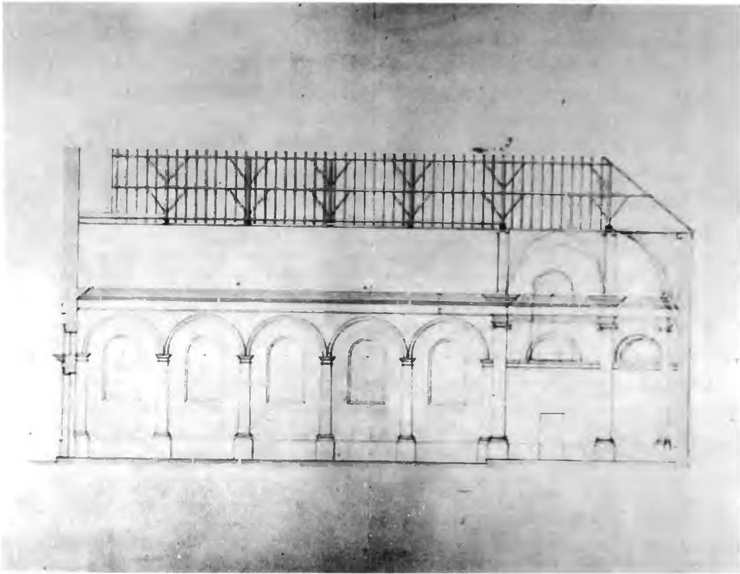
5. Overlangse doorsnede volgens het eerste ontwerp.
