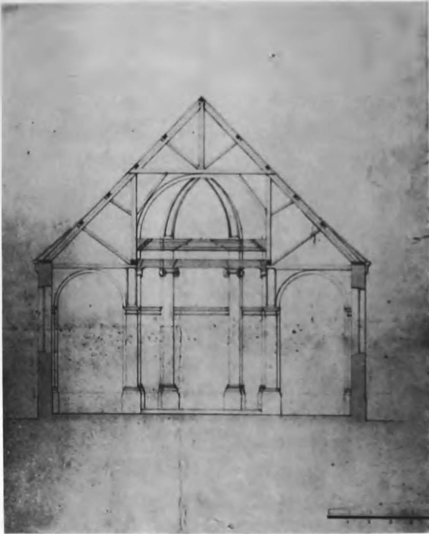
6. Dwarse doorsnede over het schip volgens het eerste ontwerp.
