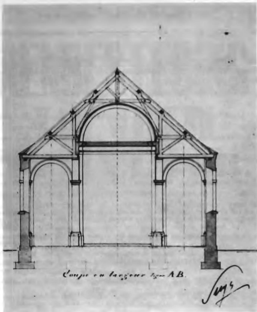
10. Dwarse doorsnede volgens het ontwerp van Suys.
