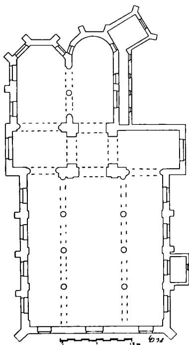
Plattegrond van de kerk te Adegem, afgebroken in 1842 : opname door arch. Minard.
