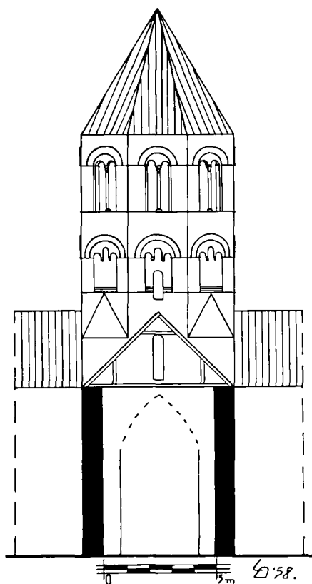
Adegem, romaanse kerk : doorsnede over het koor
